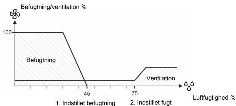
Figur 5: 1. Faldende luftfugtighed. Luftfugtigheden er under Indstillet befugning. Staldcomputeren starter befugningen. 2. Stigende luftfugtighed. Luftfugtigheden er over Indstillet fugt. Staldcomputeren øger ventilationen.
