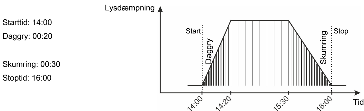
Figur 11: Normal lysdæmpning. Daggry og skumring ligger inde i lys-perioden.
