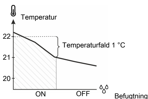
Figur 6: Faldende temperatur: Befugningen vil blive afbrudt hvis indetemperaturen er 1 °C under Indstillet temperatur. Befugningen vil ellers kunne få indetemperaturen til at falde yderligere.
