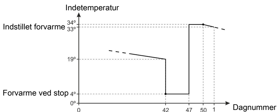
Figur 9: Eksempel på indstilling af forvarme.
