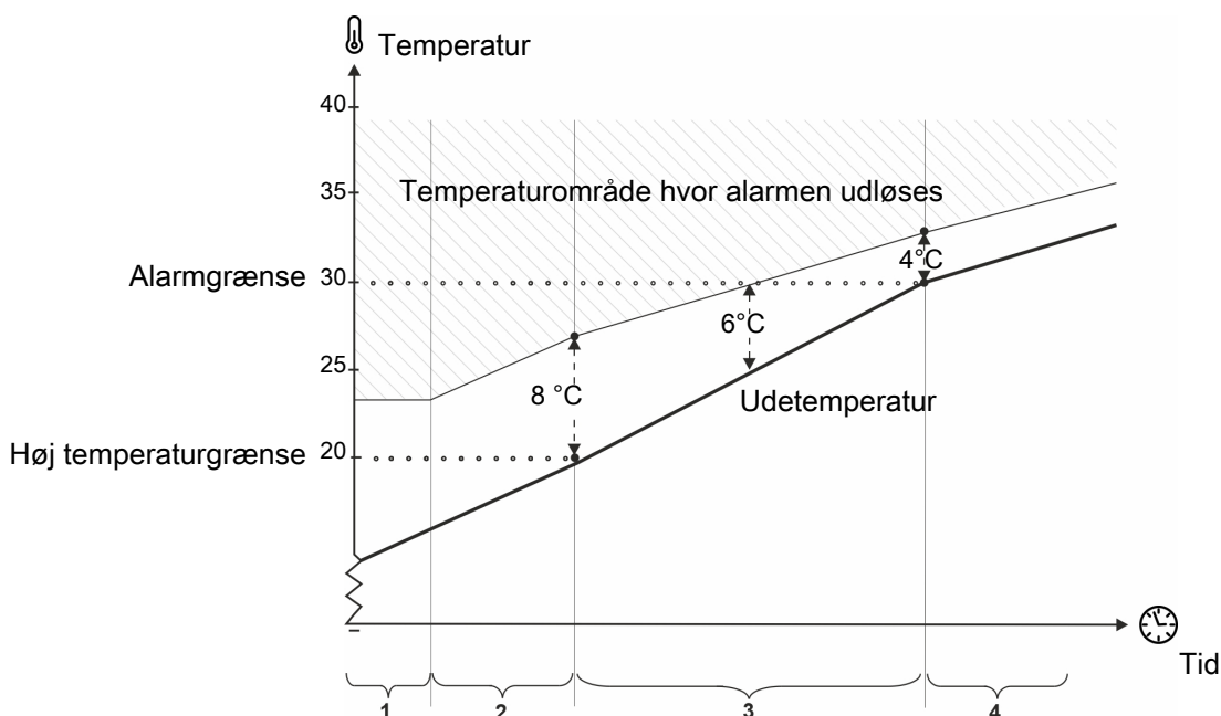
Figur 13: Sommeralarm ved 20 °C og 30 °C ude
