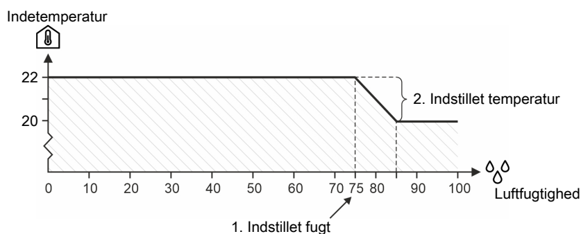
Figur 7: Fugtstyring med temperatursænkning
